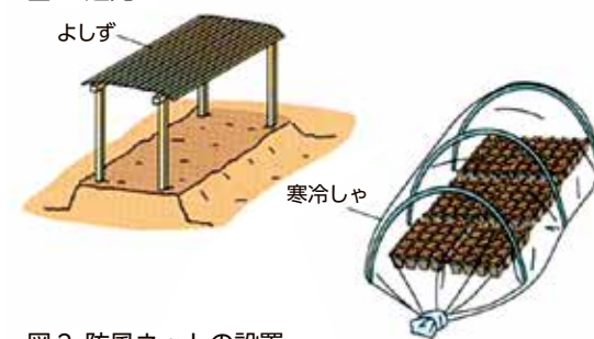
図2 防風ネットの設置
