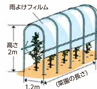
図3 雨よけ
