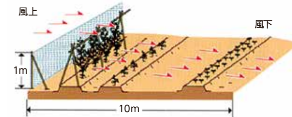
図2 防風ネットの設置
